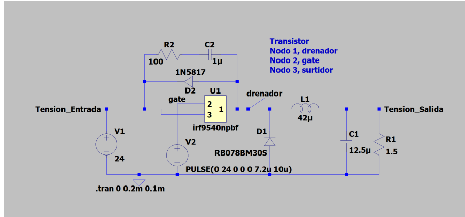
Figure 1: Circuito Simulado
